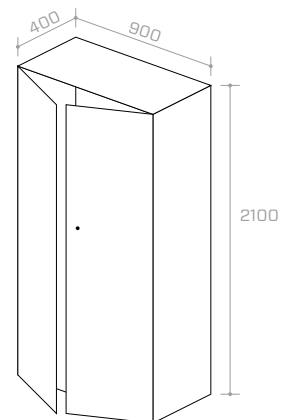
Voor liften >12 meter hefhoogte: Kast met afsluitbare deur geschikt voor binnen- en buitenopstelling
