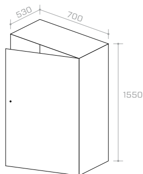
Voor liften tot 12 meter hefhoogte: Kast met afsluitbare deur geschikt voor buitenopstelling
