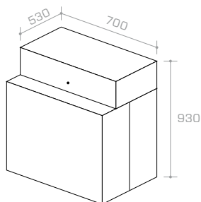
Voor liften tot 12 meter hefhoogte: Kast met deksel voor inpandige plaatsing
